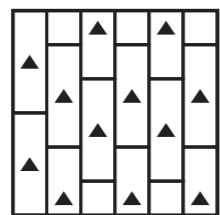
СПОСОБ УКЛАДКИ КАМЕННАЯ КЛАДКА
